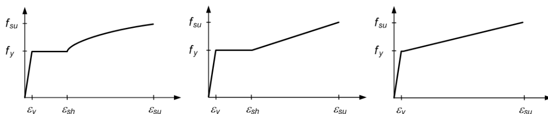
【그림 7.1】 철근의 강도 및 변형률
