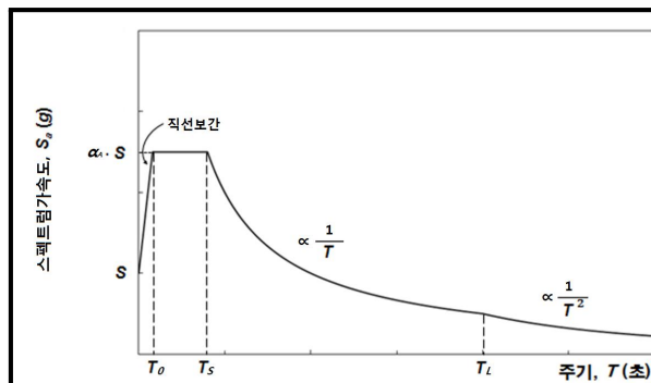
【표 9.1】 가속도표준설계응답스펙트럼 (암반지반 S1)
