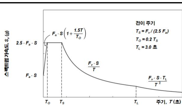
【표 9.2】 가속도표준설계응답스펙트럼 (토사지반 S2~S5)
